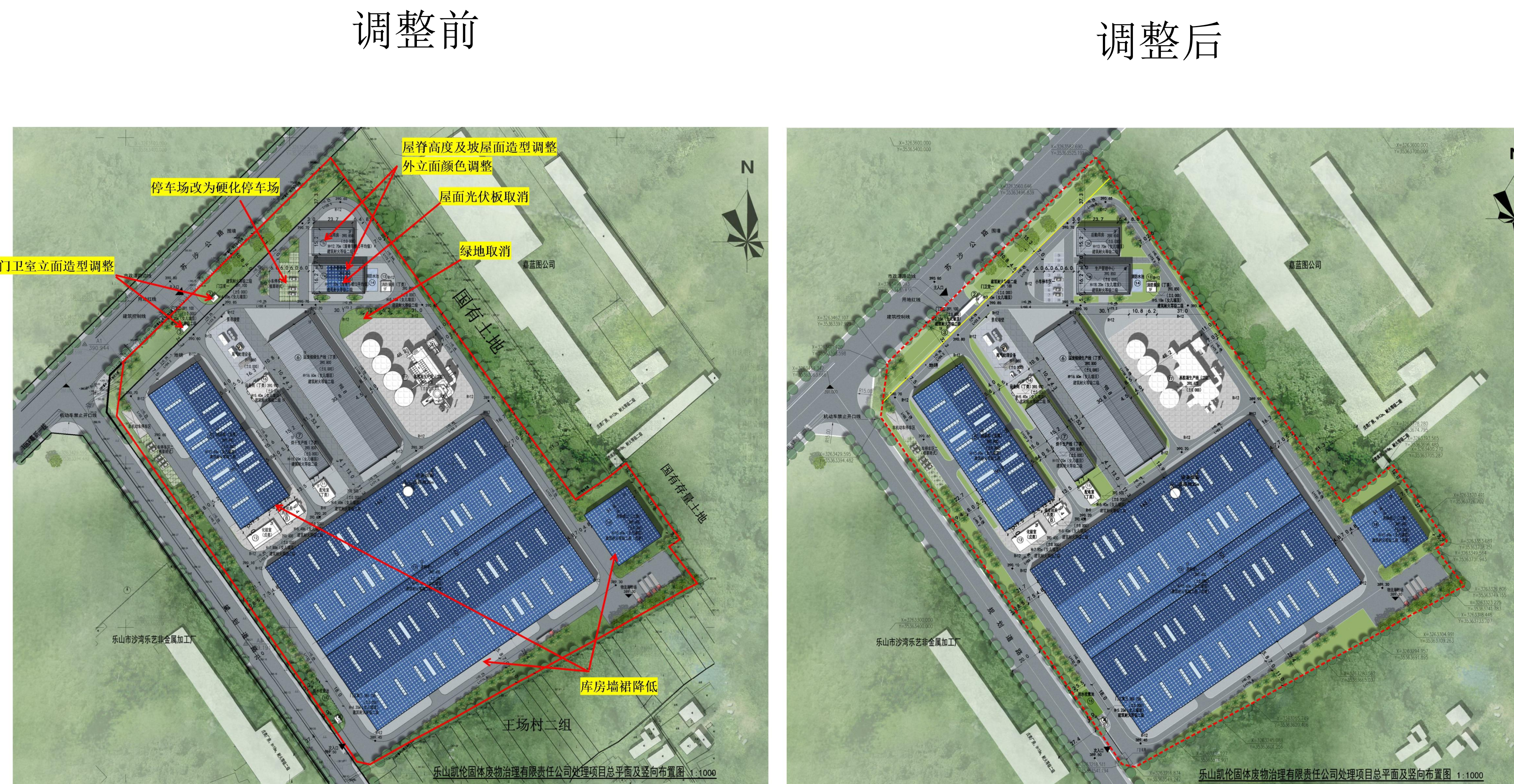
总平面对比图
