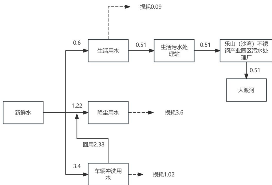
图 2-2 项目水平衡图（单位 m 3 /d）
