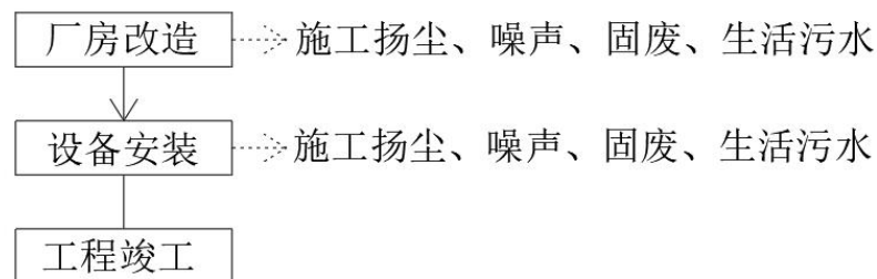
图 2-1 施工期工艺流程及产污环节图
