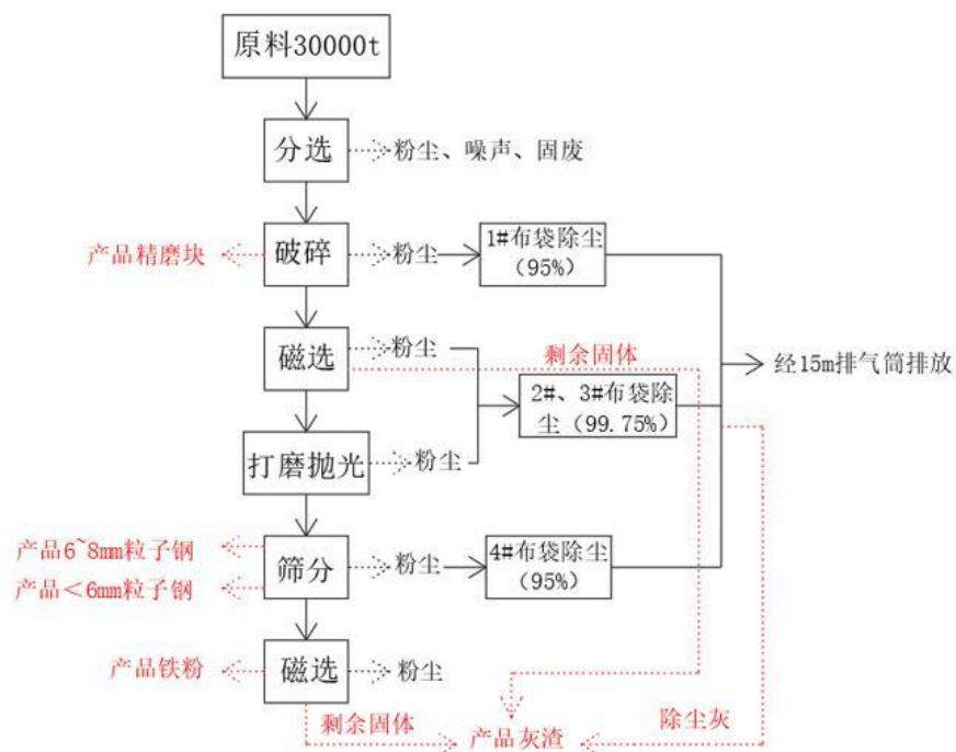
图 2-2 运营期工艺流程及产污环节图
