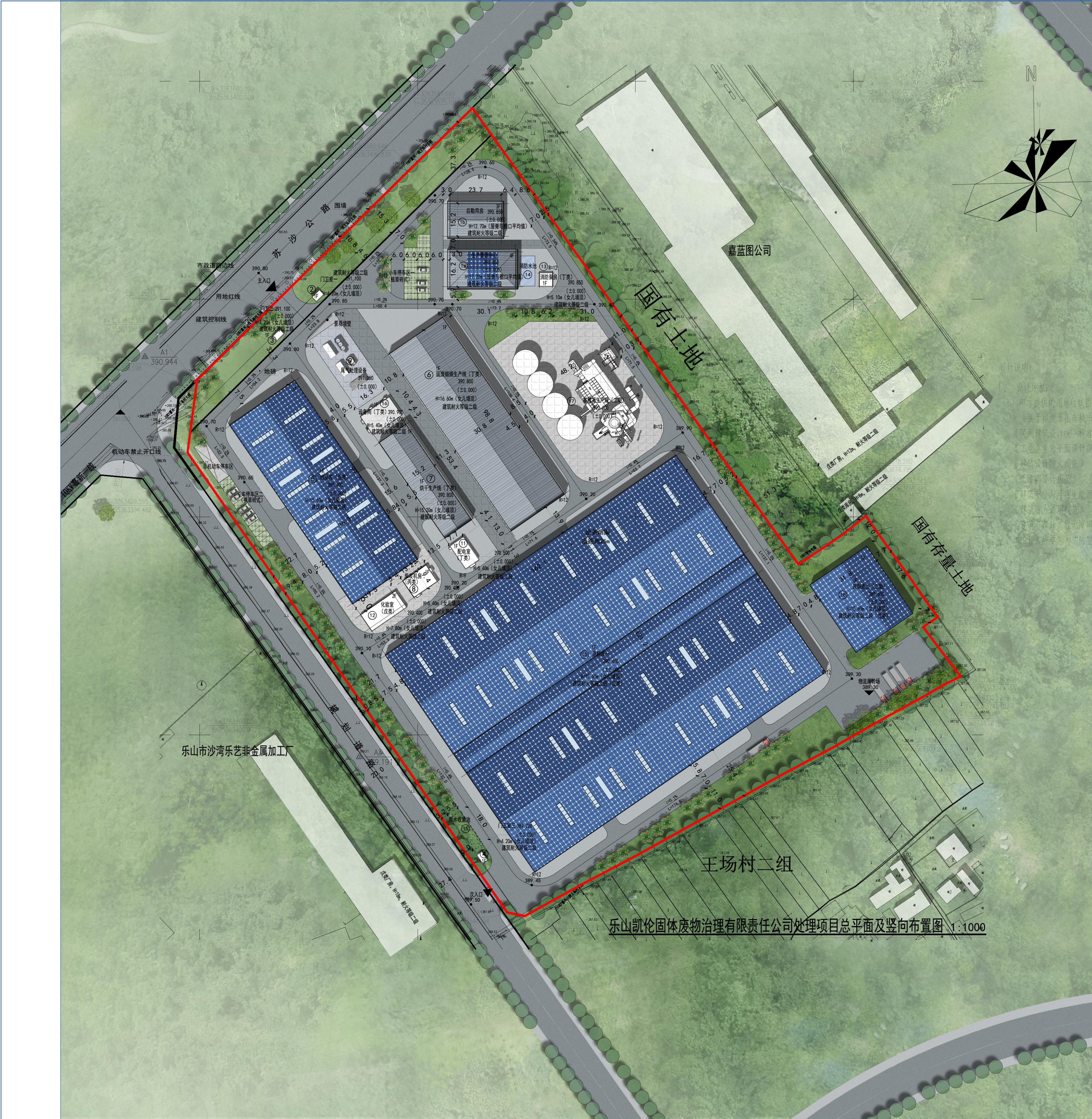
总平面图
