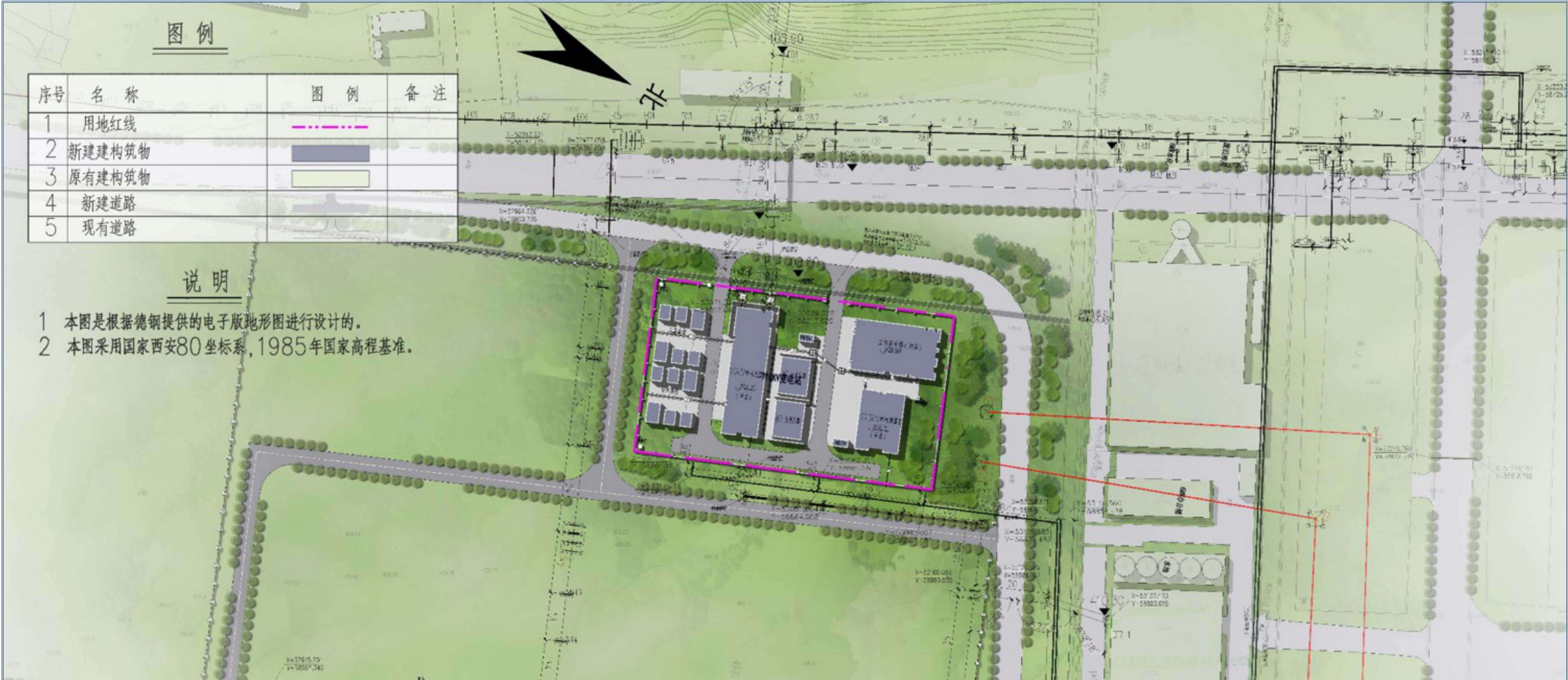
总平面图
